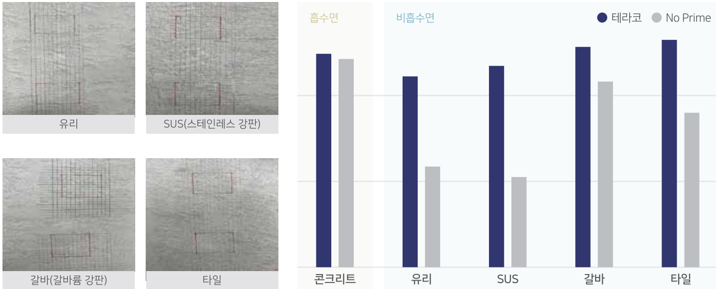
<테라본드 AP201 부착력 테스트 비교 그래프>
